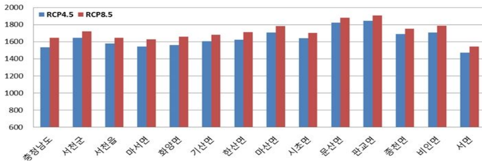
그림 3-6. 2040s의 읍면동별 연강수량 RCP 4.5(청), RCP 8.5(적)
