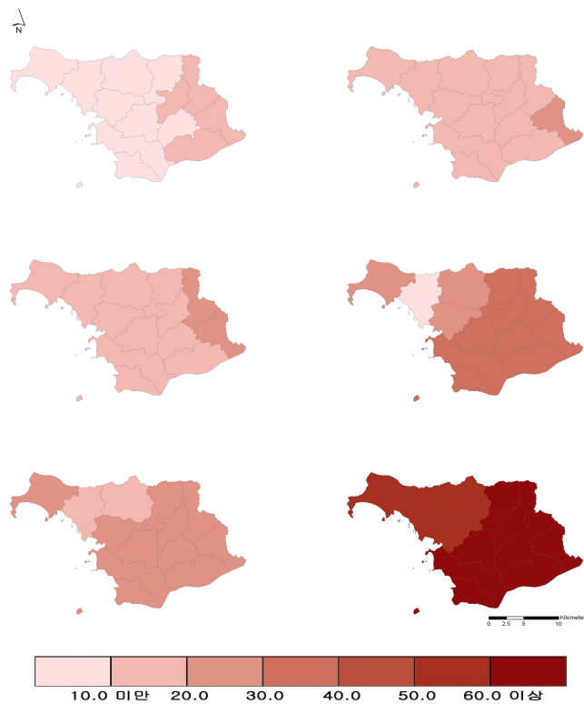
그림 3-8. RCP 4.5(좌)/8.5(우) 폭염일수 분포도 (2011~2040년(상), 2041~2070년(중), 2071~2100년(하))
