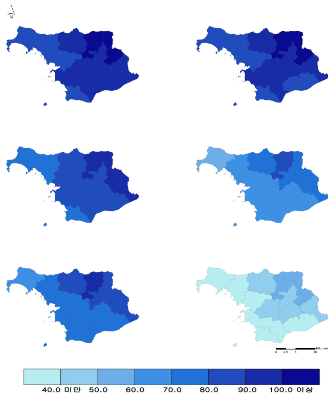
그림 3-12. RCP 4.5(좌)/8.5(우) 서리일수 분포도 (2011~2040년(상), 2041~2070년(중), 2071~2100년(하))
