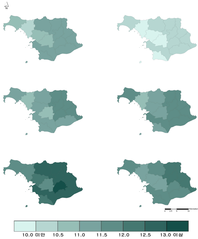
그림 3-10. RCP 4.5(좌)/8.5(우) 강수강도 분포도 (2011~2040년(상), 2041~2070년(중), 2071~2100년(하))
