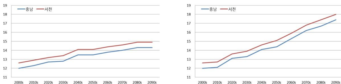
그림 3-1. 충청남도과 서천군의 평균기온 시계열 RCP 4.5(좌), RCP 8.5(우)
