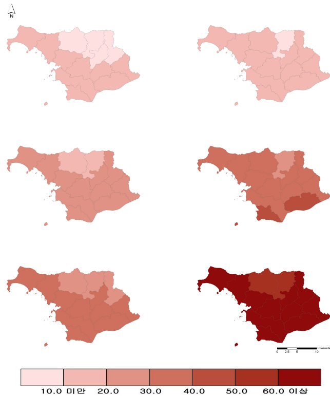
그림 3-9. RCP 4.5(좌)/8.5(우) 열대야일수 분포도 (2011~2040년(상), 2041~2070년(중), 2071~2100년(하))
