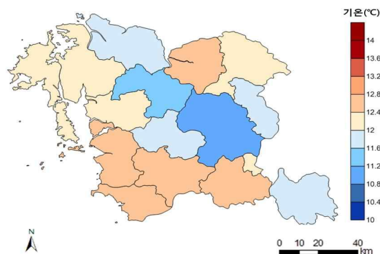
그림 2-1. 충청남도의 행정구역별 연평균기온 상세분포도(2001~2010년)
