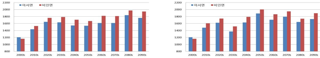
그림 3-5. 연강수량 변화폭이 가장 큰 지역과 작은 지역 RCP 4.5(좌), RCP 8.5(우)
