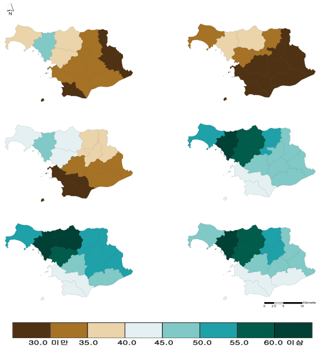
그림 3-7. RCP 4.5(좌)/8.5(우) 강수량 증가비(2001~2010년 대비 증가%) 분포도 (2011~2040년(상), 2041~2070년(중), 2071~2100년(하))
