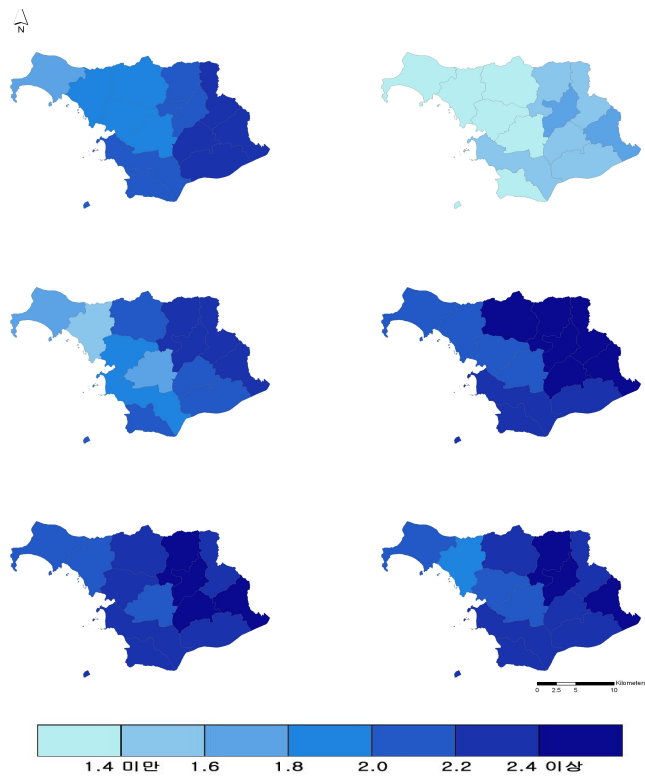
그림 3-11. RCP 4.5(좌)/8.5(우) 호우일수 분포도 (2011~2040년(상), 2041~2070년(중), 2071~2100년(하))
