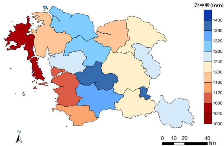
그림 2-2. 충청남도의 행정구역별 연강수량 상세분포도(2001~2010년)
