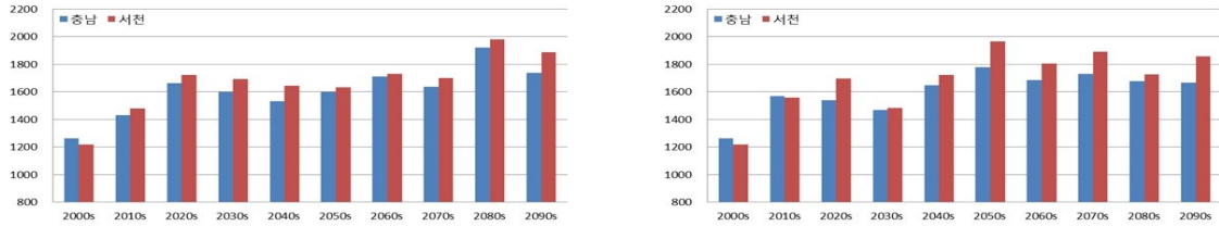
그림 3-4. 충청남도과 서천군의 연강수량 시계열 RCP 4.5(좌), RCP 8.5(우)
