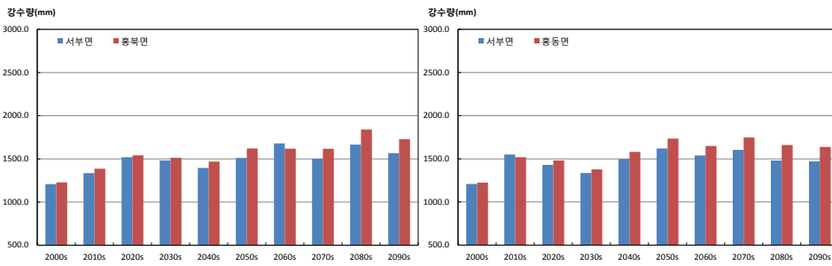
그림 3-5. 연강수량(mm) 증가율이 가장 큰 지역 (홍북면, 홍동면)과 작은 지역(서부면)의 시계열(RCP4.5(좌), RCP8.5(우))
