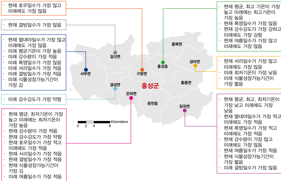
그림 5-1. 충청남도 홍성군의 읍면별 기후변화 전망 요약(RCP8.5 2071~2100년)
