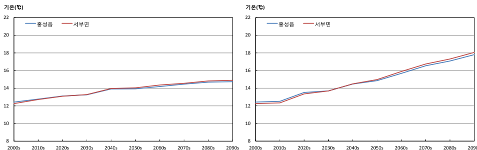
그림 3-2. 평균기온(℃) 증가율이 가장 큰 지역(서부면)과 작은 지역(홍성읍)의 시계열(RCP4.5(좌), RCP8.5(우))
