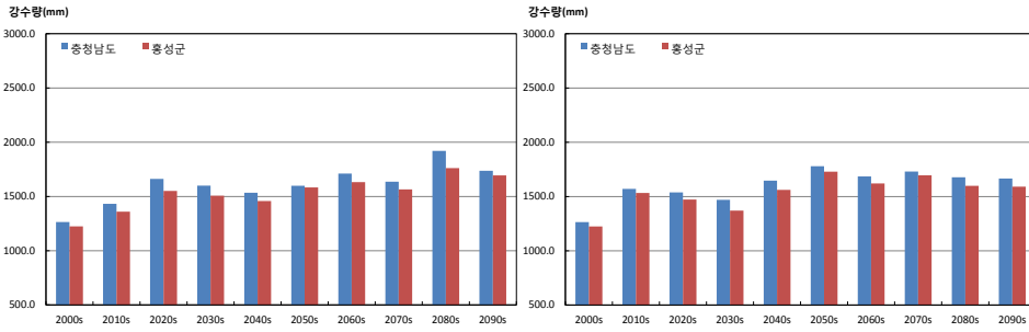
그림 3-4. 충청남도과 홍성군의 연강수량(mm) 시계열 (RCP4.5(좌), RCP8.5(우))
