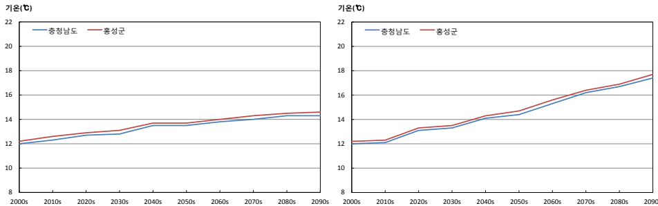
그림 3-1. 충청남도과 홍성군의 평균기온(℃) 시계열(RCP4.5(좌), RCP8.5(우))
