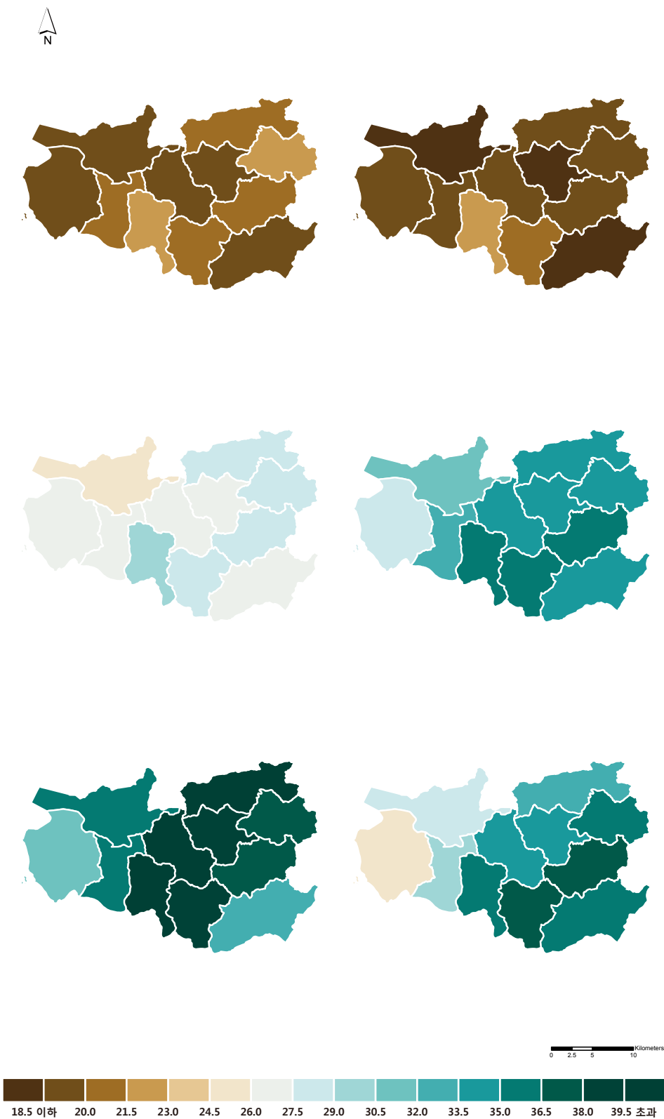
그림 3-7. 홍성군의 읍면별 강수량 증가율(%) (2001~2010년 대비) 분포도 (RCP4.5(좌)/8.5(우), 2011~2040년(상), 2041~2070년(중), 2071~2100년(하))
