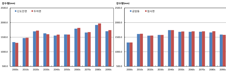
그림 3-5. 연강수량(mm) 증가율이 가장 큰 지역 (두마면, 엽사면)과 작은 지역(신도안면, 금암동)의 시계열 (RCP4.5(좌), RCP8.5(우))
