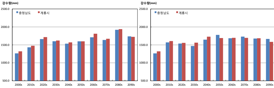
그림 3-4. 충청남도과 계룡시의 연강수량(mm) 시계열 (RCP4.5(좌), RCP8.5(우))
