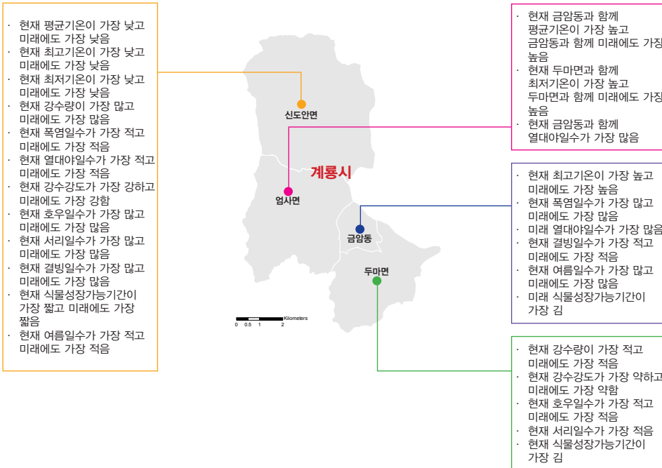
그림 5-1. 충청남도 계룡시의 면동별 기후변화 전망 요약
