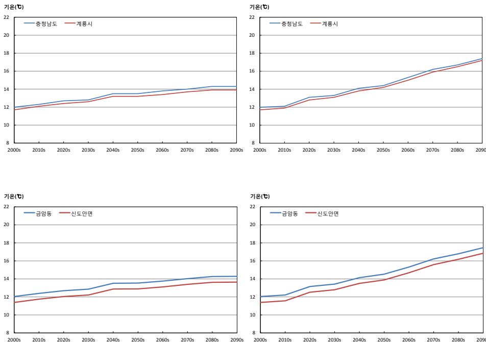
그림 3-1. 충청남도과 계룡시의 평균기온(℃) 시계열(RCP4.5(좌), RCP8.5(우))
