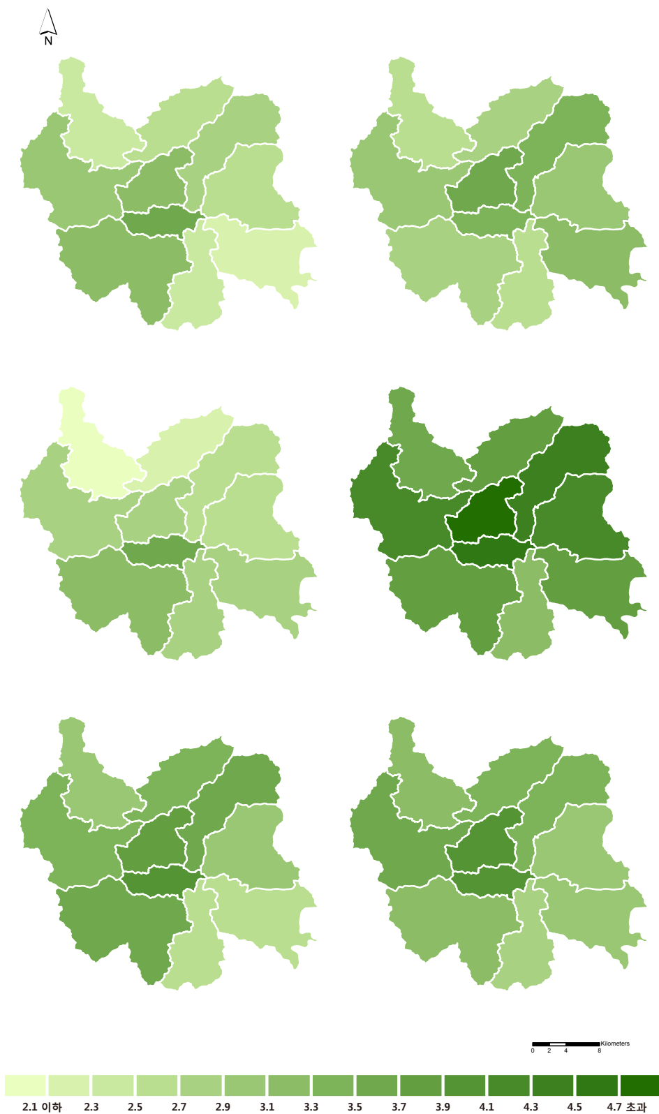
그림 3-15. 금산군의 읍면별 호우일수(일) 분포도 (RCP4.5(좌)/8.5(우), 2011~2040년(상), 2041~2070년(중), 2071~2100년(하))
