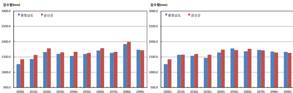
그림 3-4. 충청남도과 금산군의 연강수량(mm) 시계열 (RCP4.5(좌), RCP8.5(우))
