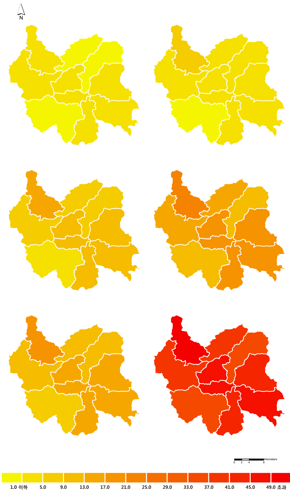
그림 3-9. 금산군의 음면별 열대야일수(일) 분포도 (RCP4.5(좌)/8.5(우), 2011~2040년(상), 2041~2070년(중), 2071~2100년(하))
