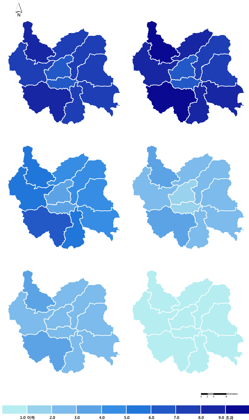
그림 3-11. 금산군의 음면별 결빙일수(일) 분포도 (RCP4.5(좌)/8.5(우), 2011~2040년(상), 2041~2070년(중), 2071~2100년(하))
