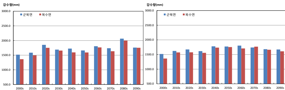
그림 3-5. 연강수량(mm) 증가율이 가장 큰 지역 (북수면)과 작은 지역(군북면)의 시계열(RCP4.5(좌), RCP8.5(우))
