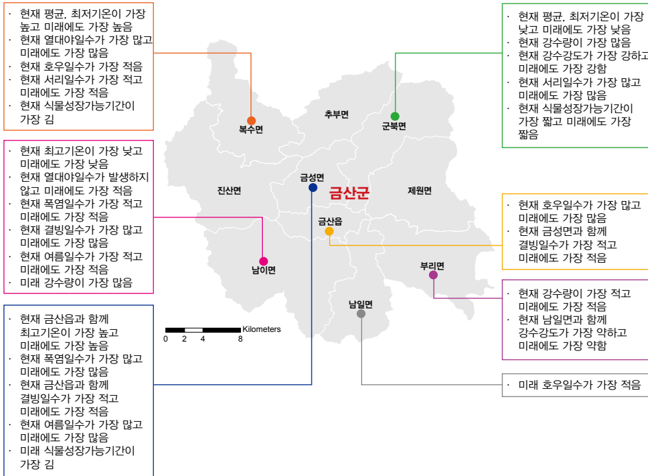
그림 5-1. 충청남도 금산군의 읍면별 기후변화 전망 요약(RCP8.5 2071~2100년)
