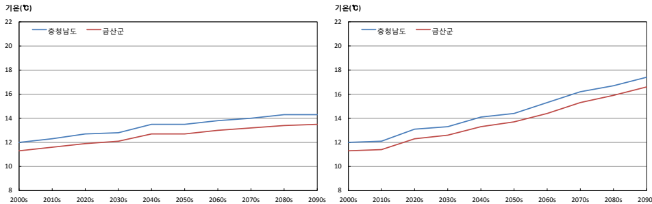
그림 3-1. 충청남도과 금산군의 평균기온(℃) 시계열(RCP4.5(좌), RCP8.5(우))
