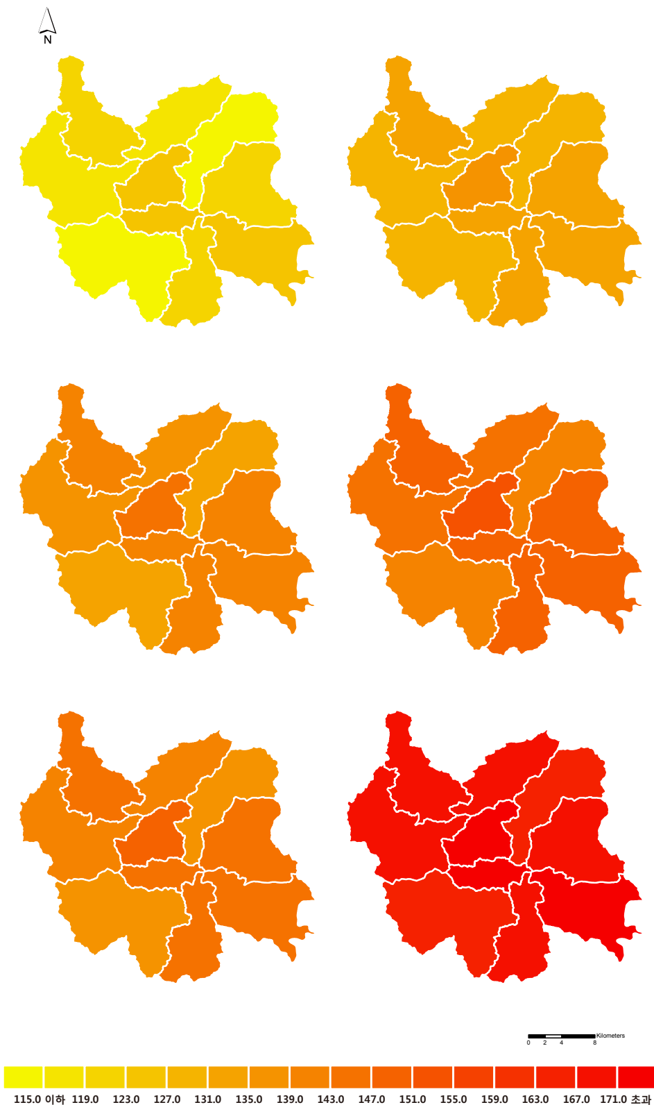
그림 3-13. 금산군의 음면별 여름일수(일) 분포도 (RCP4.5(좌)/8.5(우), 2011~2040년(상), 2041~2070년(중), 2071~2100년(하))
