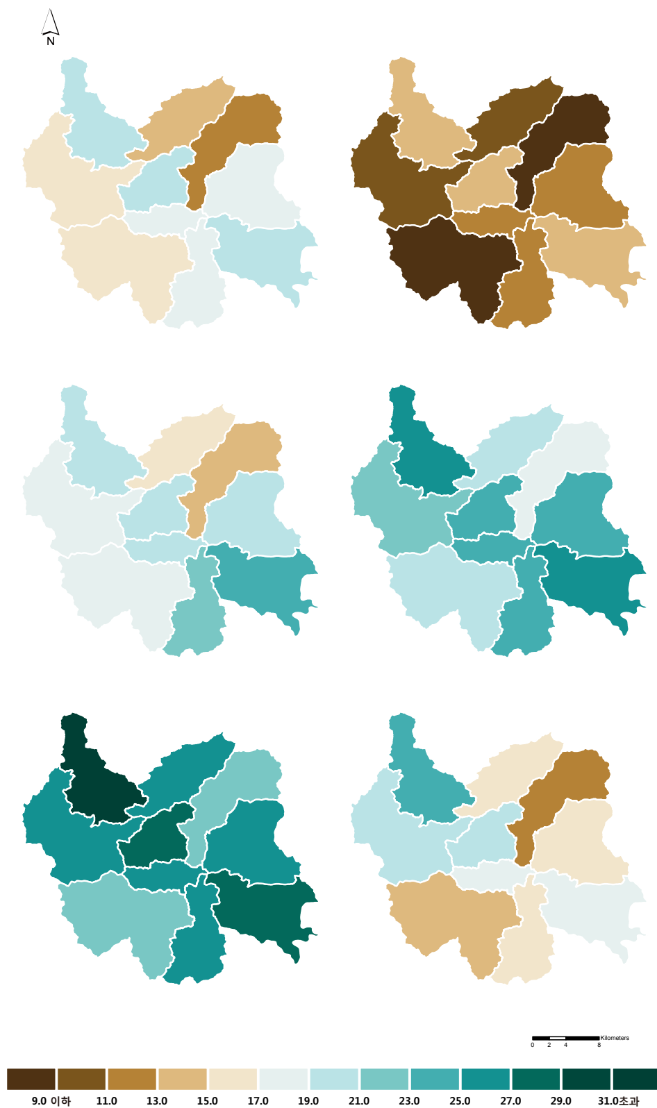
그림 3-7. 금산군의 음면별 강수량 증가율(%) (2001~2010년 대비) 분포도 (RCP4.5(좌)/8.5(우), 2011~2040년(상), 2041~2070년(중), 2071~2100년(하))
