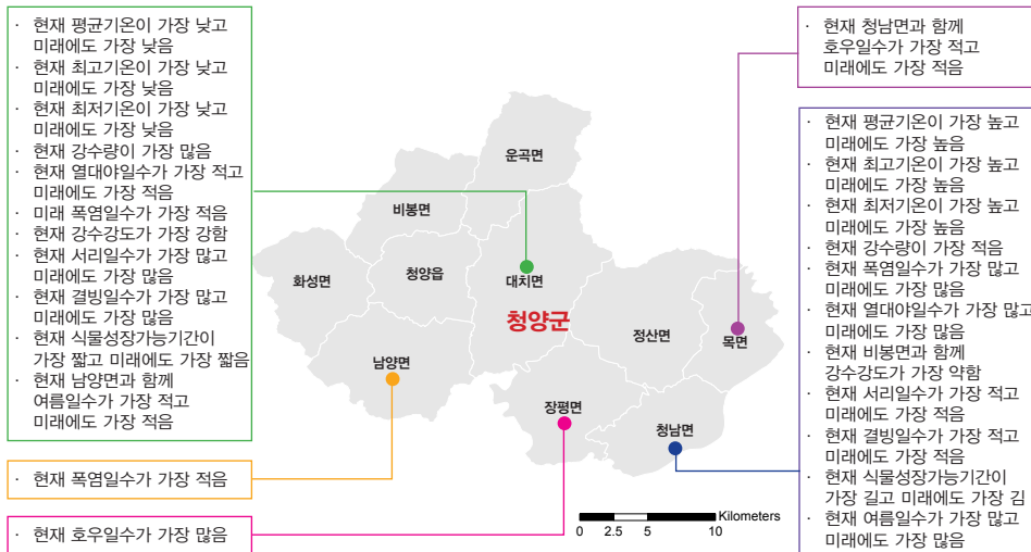
그림 5-1. 충청남도 청양군의 읍면별 기후변화 전망 요약
