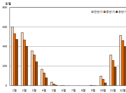
그림 4-6. 청양군의 월별 난방도일(도일) 전망 (RCP4.5(좌), RCP8.5(우))
