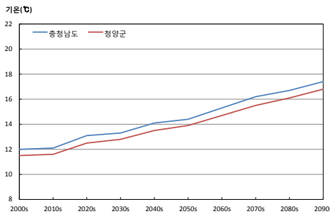
그림 3-1. 충청남도과 청양군의 평균기온(℃) 시계열(RCP4.5(좌), RCP8.5(우))
