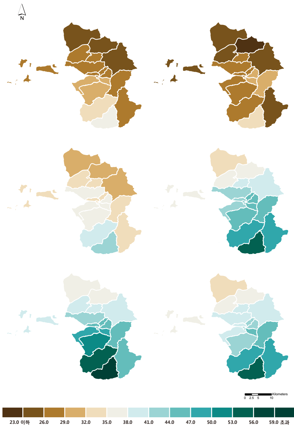
그림 3-7. 보령시의 읍면동별 강수량 증가율(%) (2001~2010년 대비) 분포도 (RCP4.5(좌)/8.5(우), 2011~2040년(상), 2041~2070년(중), 2071~2100년(하))
