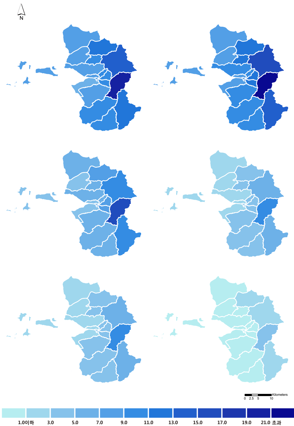
그림 3-11. 보령시의 읍면동별 결빙일수(일) 분포도 (RCP4.5(좌)/8.5(우), 2011~2040년(상), 2041~2070년(중), 2071~2100년(하))
