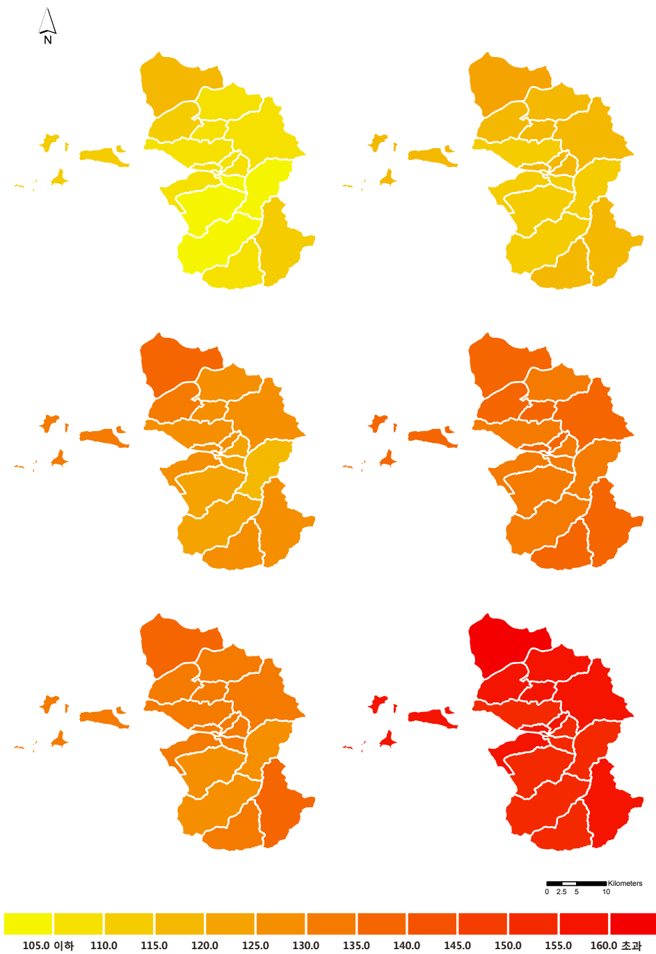
그림 3-13. 보령시의 읍면동별 여름일수(일) 분포도 (RCP4.5(좌)/8.5(우), 2011~2040년(상), 2041~2070년(중), 2071~2100년(하))
