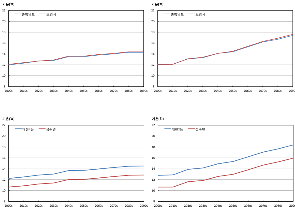
그림 3-1. 충청남도과 보령시의 평균기온(℃) 시계열(RCP4.5(좌), RCP8.5(우))
