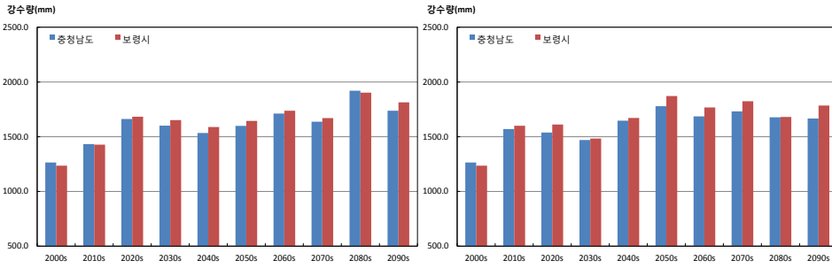
그림 3-4. 충청남도과 보령시의 연강수량(mm) 시계열 (RCP4.5(좌), RCP8.5(우))
