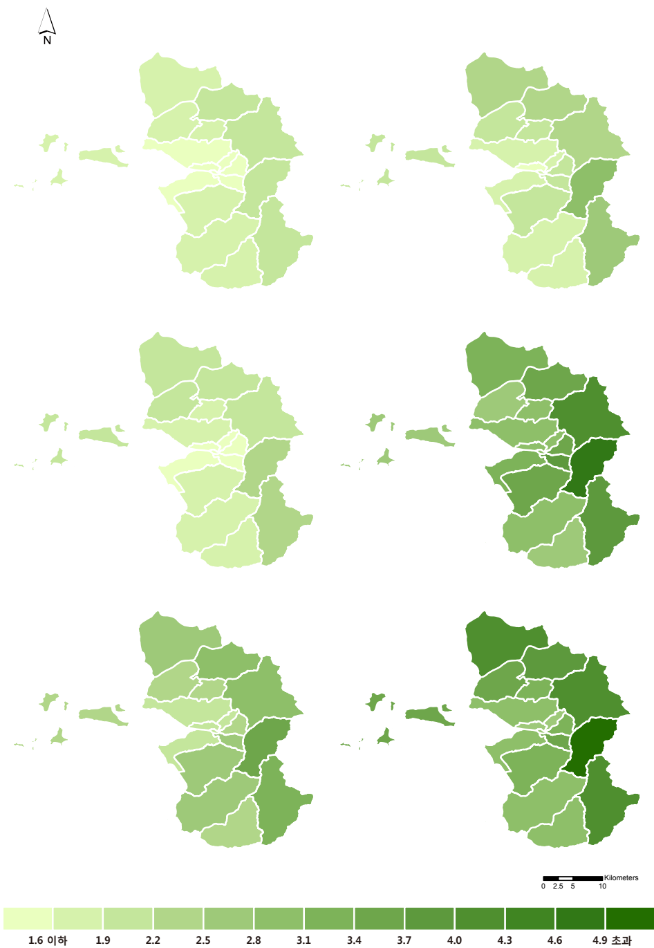
그림 3-15. 보령시의 읍면동별 호우일수(일) 분포도 (RCP4.5(좌)/8.5(우), 2011~2040년(상), 2041~2070년(중), 2071~2100년(하))
