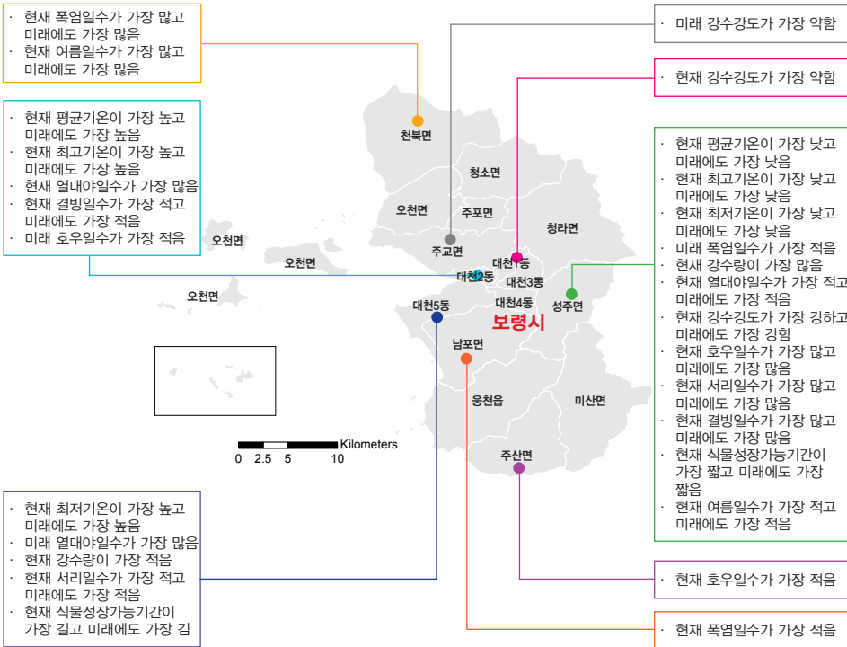
그림 5-1. 충청남도 보령시의 읍면동별 기후변화 전망 요약
