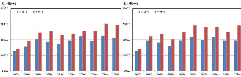
그림 3-5. 연강수량(mm) 증가율이 가장 큰 지역 (주산면)과 작은 지역(천북면)의 시계열 (RCP4.5(좌), RCP8.5(우))
