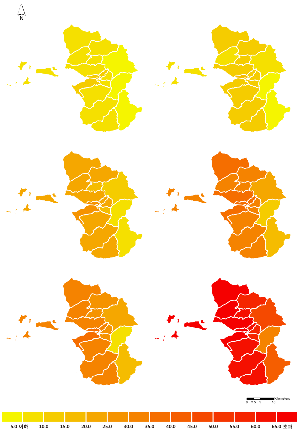
그림 3-9. 보령시의 읍면동별 열대야일수(일) 분포도 (RCP4.5(좌)/8.5(우), 2011~2040년(상), 2041~2070년(중), 2071~2100년(하))
