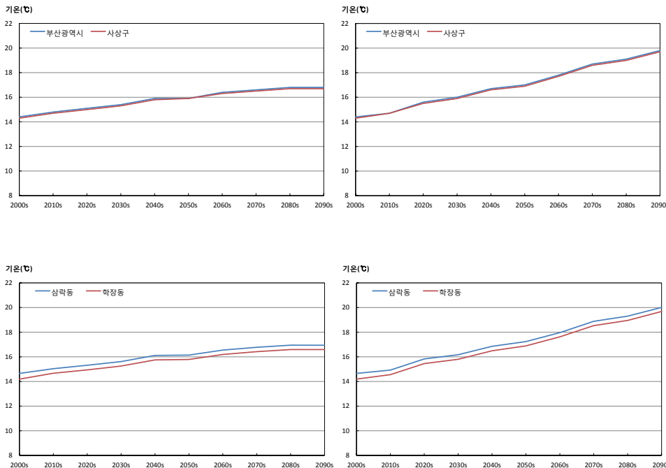
그림 3-1. 부산광역시와 사상구의 평균기온(℃) 시계열(RCP4.5(좌), RCP8.5(우))
