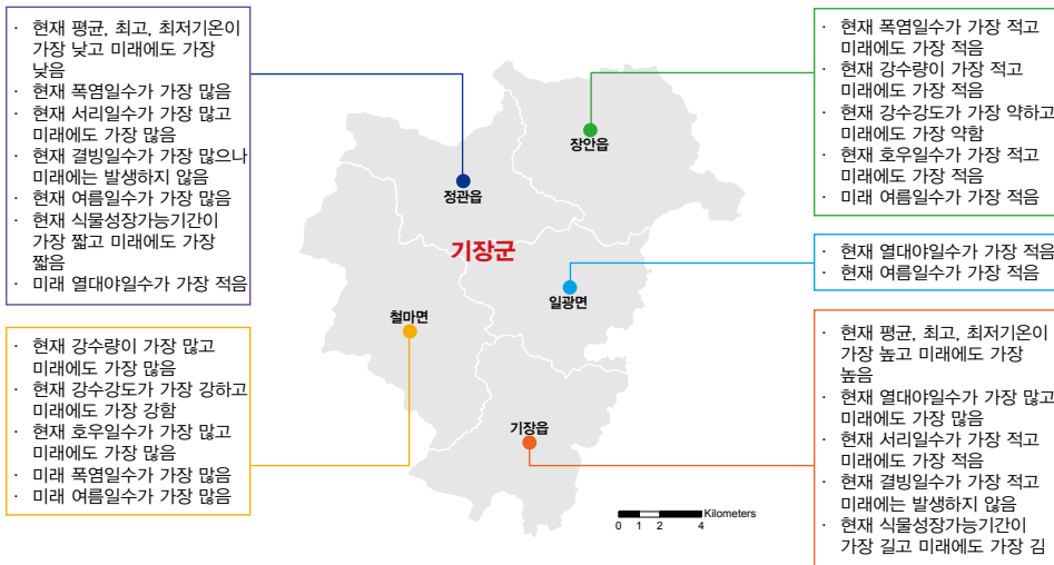
그림 5-1. 부산광역시 기장군의 음면별 기후변화 전망 요약(RCP8.5 2071~2100년)
