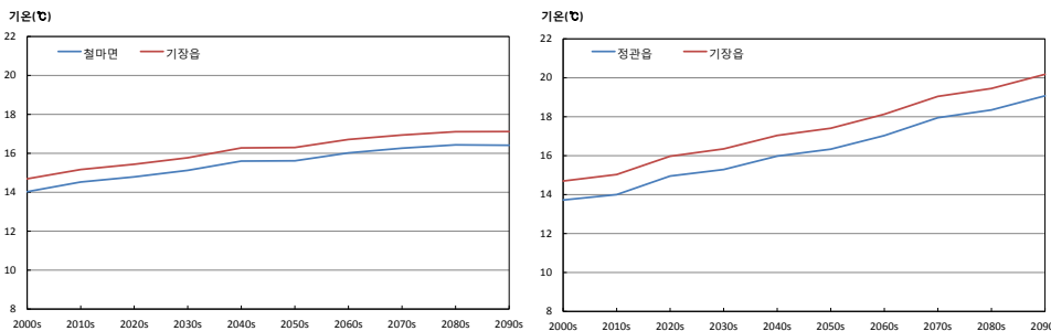
그림 3-2. 평균기온(℃) 증가율이 가장 큰 지역(기장읍)과 작은 지역(철마면, 정관읍)의 시계열(RCP4.5(좌), RCP8.5(우))
