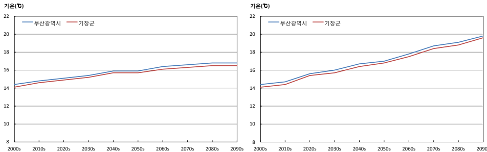
그림 3-1. 부산광역시와 기장군의 평균기온(℃) 시계열(RCP4.5(좌), RCP8.5(우))
