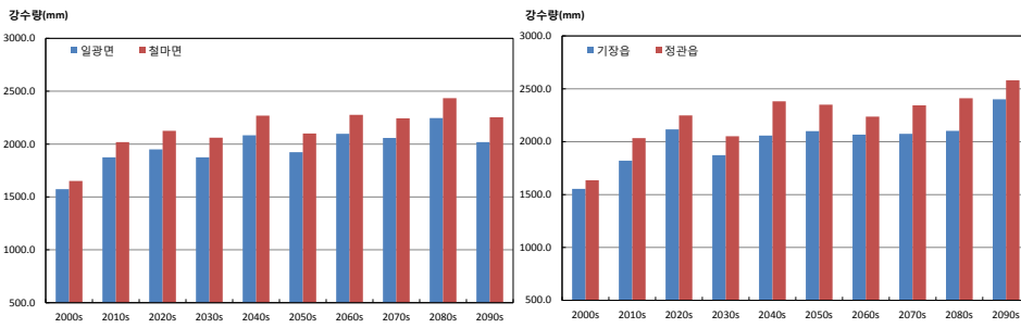
그림 3-5. 연강수량(mm) 증가율이 가장 큰 지역(철마면, 정관읍)과 작은 지역(일광면, 기장읍)의 시계열(RCP4.5(좌), RCP8.5(우))
