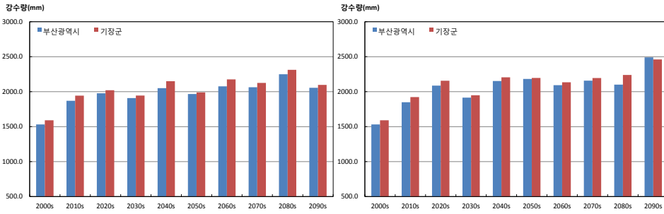
그림 3-4. 부산광역시와 기장군의 연강수량(mm) 시계열 (RCP4.5(좌), RCP8.5(우))
