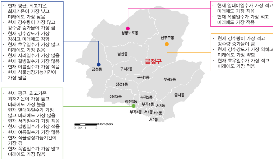
그림 5-1. 부산광역시 금정구의 동별 기후변화 전망 요약
