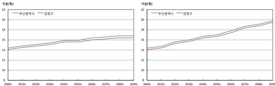
그림 3-1. 부산광역시와 금정구의 평균기온(℃) 시계열(RCP4.5(좌), RCP8.5(우))
