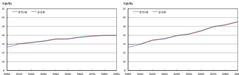
그림 3-2. 평균기온(℃) 증가율이 가장 큰 지역(금성동)과 작은 지역(장전2동)의 시계열(RCP4.5(좌), RCP8.5(우))
