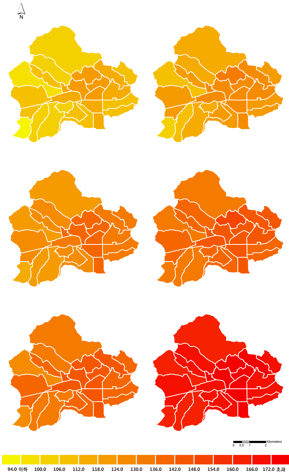
그림 3-13. 부산진구의 동별 여름일수(일) 분포도 (RCP4.5(좌)/8.5(우), 2011~2040년(상), 2041~2070년(중), 2071~2100년(하))
