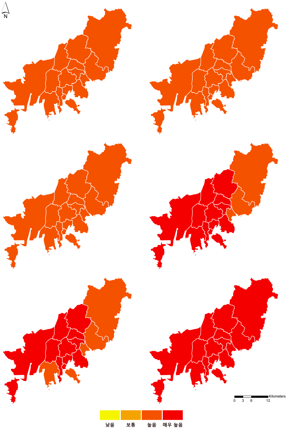
그림 4-4. 부산광역시 구군별 불해지수 분포도 (RCP4.5(좌)/8.5(우), 2011~2040년(상), 2041~2070년(중), 2071~2100년(하))
