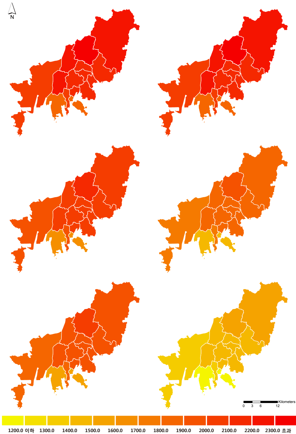
그림 4-8. 부산광역시 구군별 난방도일(도일) 분포도 (RCP4.5(좌)/8.5(우), 2011~2040년(상), 2041~2070년(중), 2071~2100년(하))
