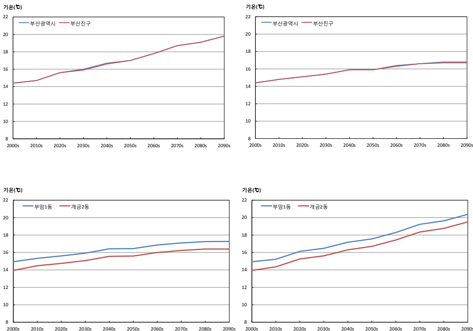
그림 3-1. 부산광역시와 부산진구의 평균기온(℃) 시계열(RCP4.5(좌), RCP8.5(우))
