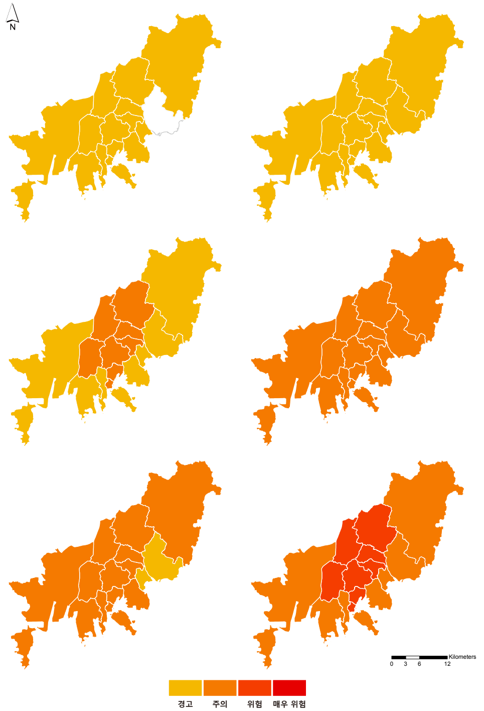
그림 4-3. 부산광역시 구군별 열지수 분포도 (RCP4.5(좌)/8.5(우), 2011~2040년(상), 2041~2070년(중), 2071~2100년(하))
