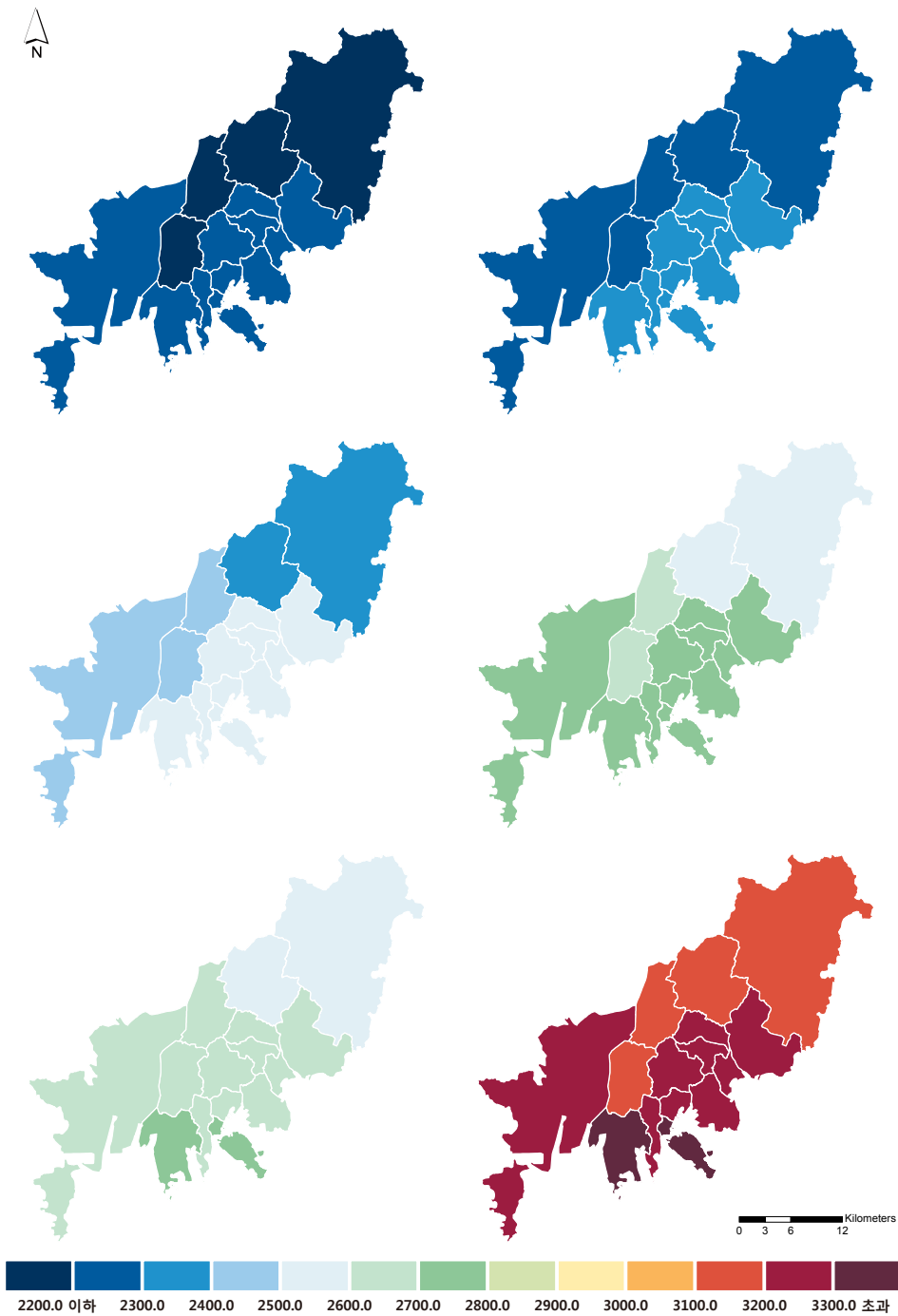
그림 4-2. 부산광역시 구군별 유효적산온도(10℃)(℃) 분포도 (RCP4.5(좌)/8.5(우), 2011~2040년(상), 2041~2070년(중), 2071~2100년(하))
