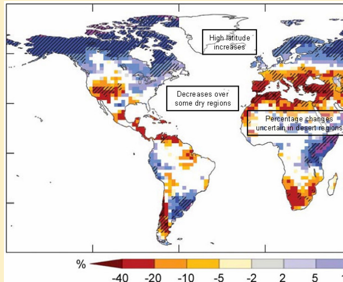
그림 3.5. 1980~1999년 대비 2090~2099년 연간 유출량(물 가용성 %)의 상대적 변화. 모델의 중간값이다. 하얗게 보이는 지역은 12개 모델에서 변화의 부호가 66% 미만 일 90% 이상 일치하는 지역이다. 20세기 대범위 유출량 관측치의 시뮬레이션 품질은 다르다. 전지구 연간 유출량 지도는 넓은 범위에 대해 표현한 것으로, 그보다 강우량과 유출량이 매우 적은 지역(예: 사막)에서는 강우량이 조금만 변해도 %로는 변화 전망의 부호와 최근에 관측된 경향이 일치하지 않는다. 유출량이 증가할 것으로 유출량 감소 같은 서로 다른 계절적 효과가 예상된다. 여기 제시한 것과 상당히 다른 그림 3.4, 그림 SYR 3.3의 가정과 통하도록 조정하였음. WG II 3.3.1, 3.4.1, 3.5.1)
