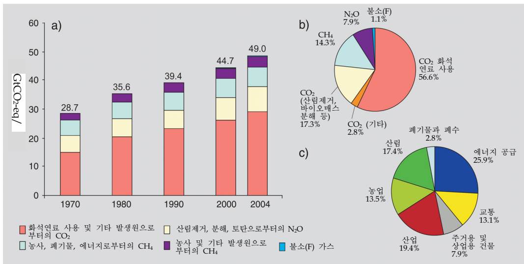
그림 2.1. (a) 1970~2004년 지구 전체 인위적 온실가스 연간 배출량. (b) 2004년 인위적 온실가스 총 배출량 중 가스별 배출량(CO 2 -상당). (c) 2004년 인위적 온실가스 총 배출량 중 부문별 배출량(CO 2 -상당). (산림에는 산림제거 포함). {WG III 그림 TS 1a, TS 1b, TS 2b}
