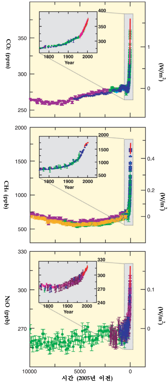
그림 2.3. 대기 중 CO 2 , CH 4 , N 2 O의 지난 10,000년 동안(큰 패널)과 1750년 이후(삽입된 패널)의 농도, 빙핵(각 연구별로 기호에 다른 색을 사용)과 대기 샘플(붉은선)을 분석한 데이터를 사용했다. 큰 패널의 오른쪽 Y축은 1750년 대비 복사강제력을 나타낸다. {WG I 그림 SPM.1}
