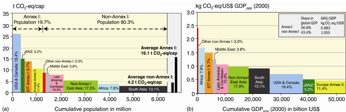
그림 2.2. (a) 2004년에 국가 그룹의 인구에 따른 1인당 온실가스 배출량의 지역적 분포(국가그룹에 대한 정의는 부록 참고). (b) 2004년에 국가 그룹의 GDP에 따른 GDP ppp 1달러(US$) 당 온실가스 배출량의 지역적 분포. 막대 안의 %는 전지구 온실가스 배출량에서 그 지역이 차지하는 비율을 뜻한다. {WG III 그림 SPM.3A, SPM.3B}
