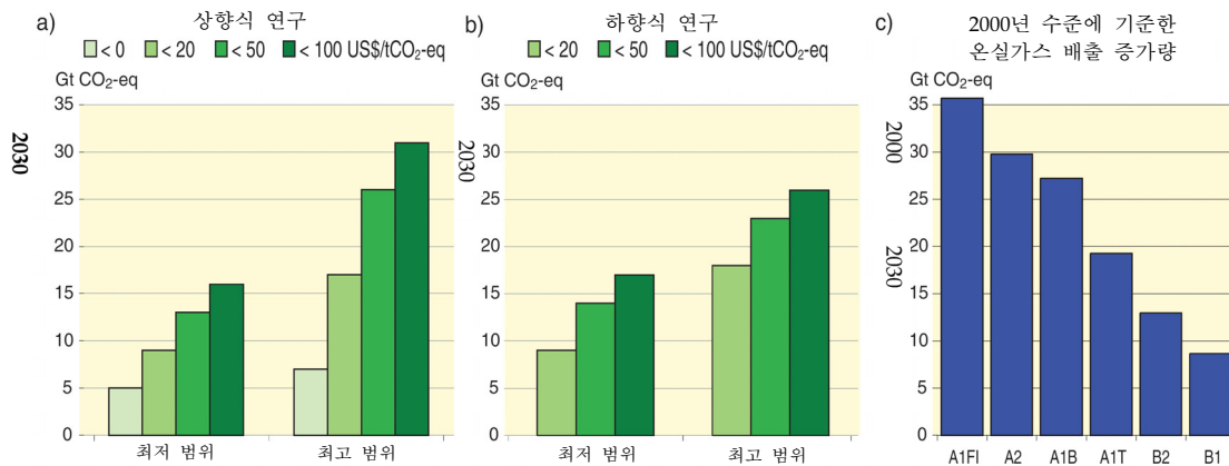
그림 4.1. 상향식 연구(a)와 하향식 연구(b)에서 추정된 2030년 전지구 경제적 완화 잠재력과 SRES 시나리오에 따른 2000년 온실가스 배출량 (40.8 GtCO 2 상당/yr)(c) 대비 2030년의 배출량 증가 전망. 주: 2000년의 온실가스 배출량에 지상 바이오매스의 부식에 따른 배출량은 포함되어 있지 않다. 목재로 베어나가거나 벌채된 후에 남아있고 토탄 연소와 토탄토양의 배수를 통해 배출되는 바이오매스는 SRES 시나리오와의 일관성을 유지하기 위해 제외되었다. {WG III 그림 SPM.4, SPM.5A, SPM.5B}
