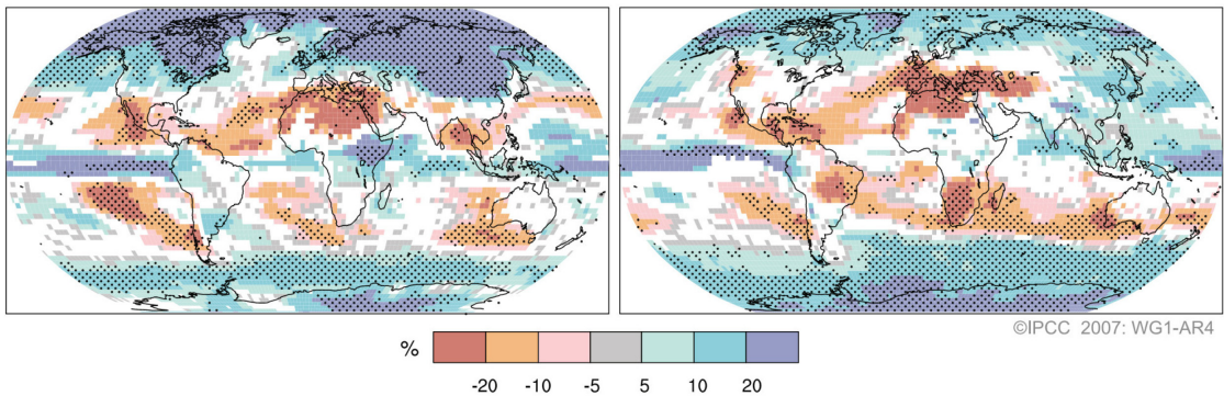
그림 3.3. 1980~1999년 대비 2090~2099년 강수의 상대적 변화(%). 값들은 SRES A1B 시나리오에 기초한 12~20월(좌측)과 6~8월(우측)의 다중 모델 평균이다. 하얗게 보이는 부분은 모델들에서 변화의 부호가 66% 미만 일치하는 지역이고, 조밀한 점들로 표현된 부분은 90% 이상 일치하는 지역이다.
