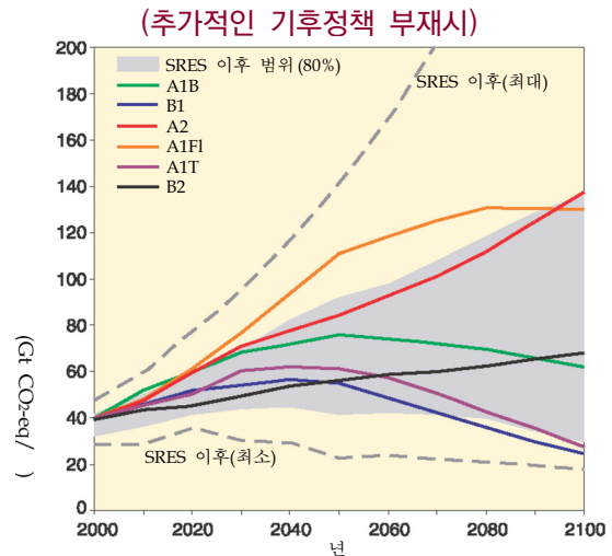
그림 3.1. 추가 기후정책이 없을 때의 전지구 온실가스 배출량(CO 2 -상당/yr) 전망. 유색 실선은 SRES 마커 시나리오 6가지, 회색 음영은 SRES 이래 발표된 최근 시나리오들(SRES 이후 시나리오들)의 80 백분위수(퍼센타일) 범위를 나타낸다. 점선은 SRES 이후 시나리오의 전체 범위를 나타낸다. 배출량은 CO 2 , CH 4 , N 2 O, F-가스의 배출량이다. {WG III 1.3, 3.2, 그림 SPM.4}
