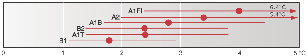
비완화 시나리오에서 1980~1999년 대비 2090~2099년의 온난화
