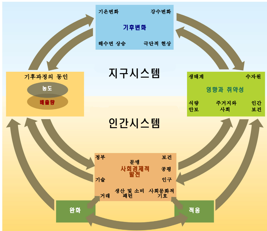
그림 1.1 기후변화의 인위적 동인(drivers)과 영향, 기후변화에 대한 대응 및 이들의 관계
