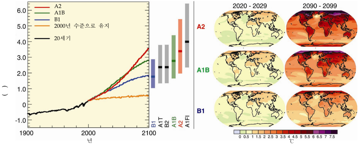
그림 3.2. (좌): 실선은 SRES 시나리오 A2, A1B, B1에 따른 지표 온난화(1980~1999년 대비)의 다중 모델 지구 평균을 20세기 시뮬레이션에 연장시켜 나타낸 것이다. 오렌지색 실선은 농도를 2000년 수준으로 일정하게 유지한 실험의 결과이다. 그림의 중앙에 있는 막대는 6가지 SRES 마커 시나리오에 대해 평가된 1980~1999년 대비 2090~2099년의 최적 추정치(각 막대의 실선)와 가능한 범위를 나타낸다. 막대의 최적 추정치와 가능한 범위는 그림의 왼쪽에 있는 AOGCM 뿐 아니라 독립된 모델 및 관측치 제약의 결과를 포함시켜 평가되었다. (우): 1980~1999년 대비 21세기 초기와 말기의 지표 기온 변화 전망. SRES 시나리오 A2(위), A1B(가운데), B1(아래)에 대하여 2020~2029(좌측)년 10년과 2090~2099년(우측)10년을 평균한 다중 AOGCM의 평균 전망이다.
