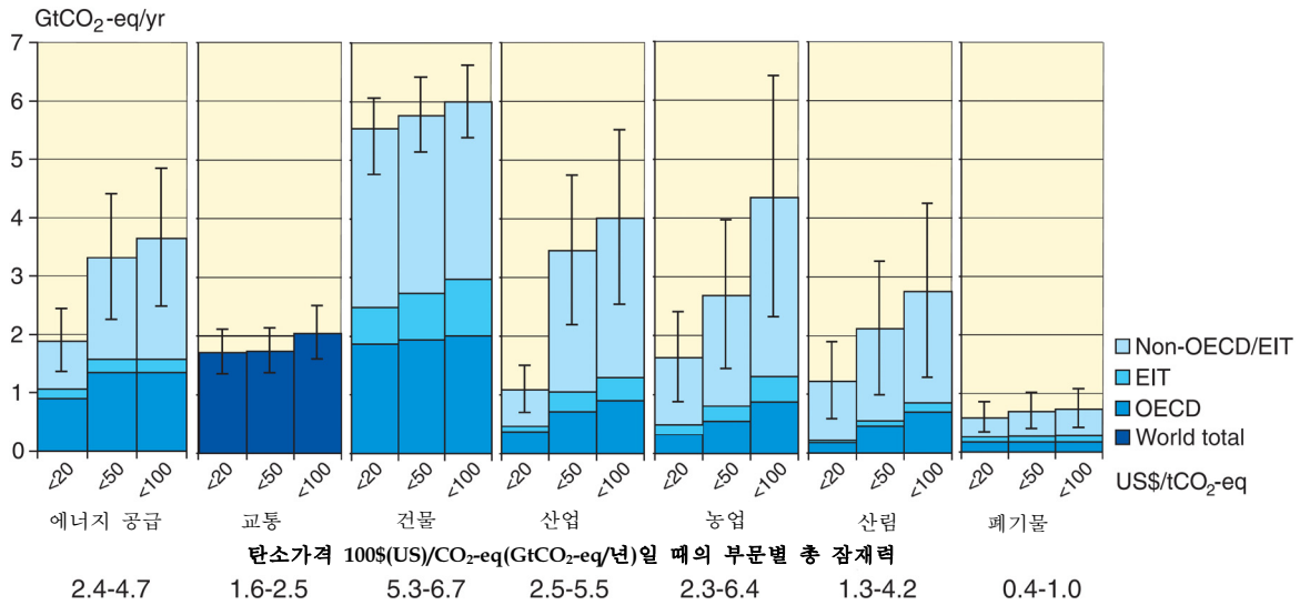
그림 4.2. 상향식 연구에서 도출된 2030년 부문별 경제적 완화 잠재력 추정치. 이 잠재력에는 생활방식 변화 같은 기술 외적인 옵션은 포함되어 있지 않다. {WG III 그림 SPM.6}
