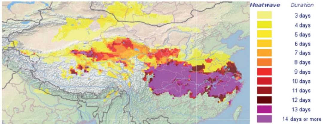
[그림 2-3-17] 2022년 중국지역 폭염지속기간(일). 노란색에서 보라색으로 갈수록 지속기간은 길어지는 것을 의미함 (출처: 유럽연합 지구관측소)
