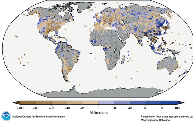
[그림 2-3-18] 2022년 6월 강수 편차 분포도 (출처: NOAA)
