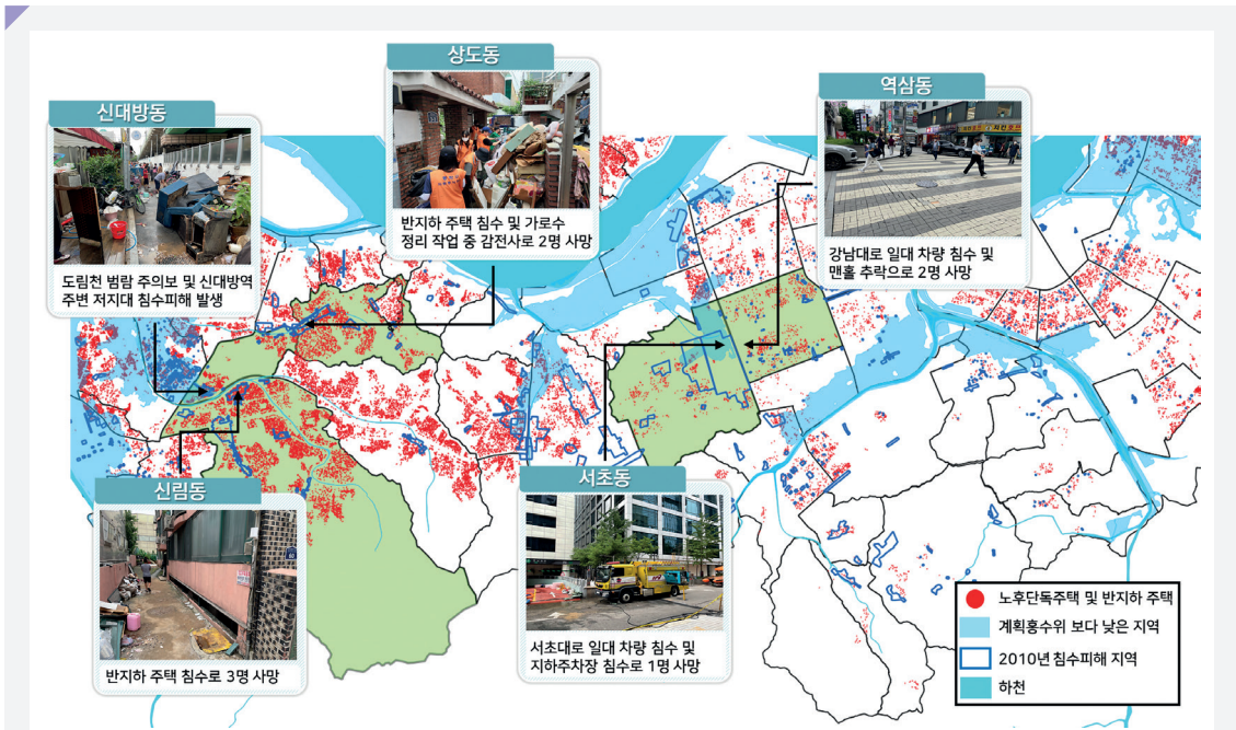
[그림 3-6-2] 2022년 8월 8일 서울시 침수피해 현황 및 취약요소 분포 (출처: 김준성 외, 2022. “기후위기시대 도시침수 예방대책: 2022년 수도권 집중호우의 교훈”)
