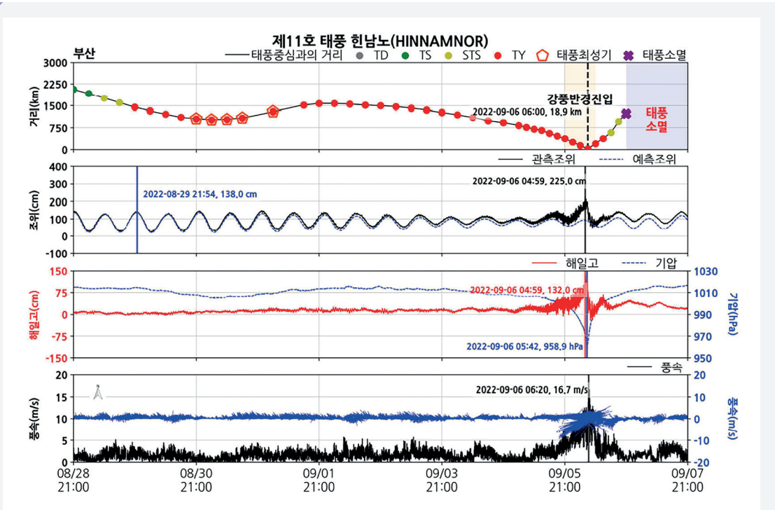
[그림 3-2-10] 제11호 태풍 ‘힌남노(HINNAMNOR)’ 통과시 부산 조위관측소에서의 해일고 및 기상자료 시계열 (그림출처: 국립해양조사원 2022 Vol. 3 ‘태풍분석보고서’)
