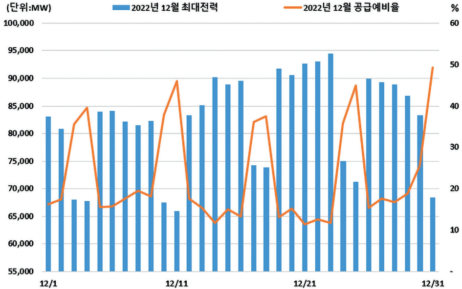
[그림 3-7-2] 2022년 12월 일별 최대전력 및 공급 예비율 (출처: 전력통계정보시스템(episis.kpx.or.kr) '최대전력수급' 자료 활용)
