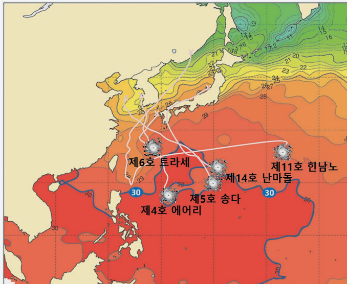
[그림 2-2-4] 2022년 영향 태풍 경로도
