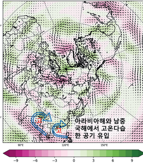
[그림 2-3-19] 2022년 6월 평균 지상 바람 편차 분포도 (출처: 기상청)
