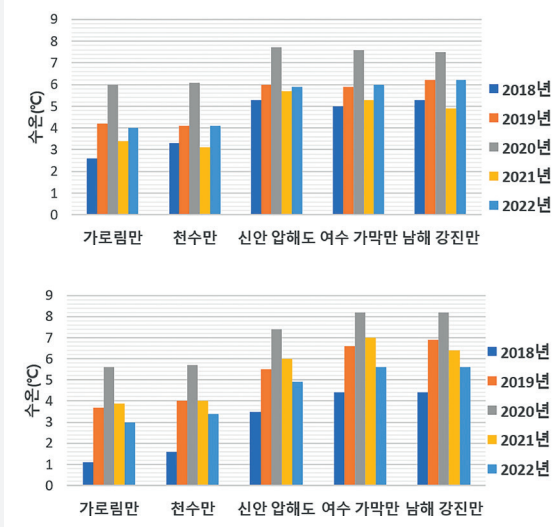
〈 주요 저수온 발생해역의 최근 5년간 월평균 표층수온 비교(1~2월) 〉
