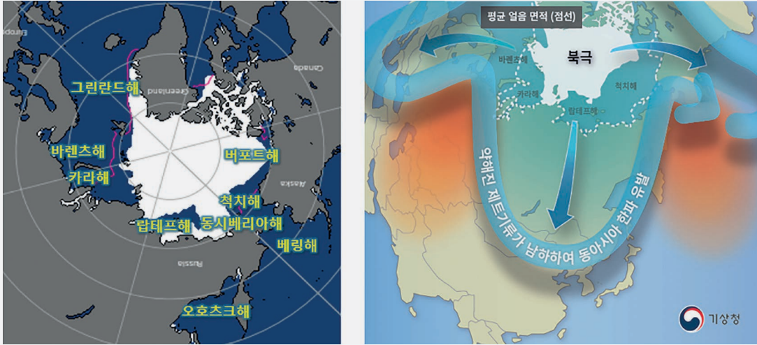
[그림 2-3-4] (왼쪽)2022년 10월 북극 해빙면적, (오른쪽)바렌츠-카라해의 해빙면적이 적은 경우, 동아시아 지역 한파 영향 모식도 ※ (왼쪽) 출처: 미국 설빙국립센터(NSIDC), 분홍색 선: 10월 북극 해빙 평년(1981~2010) 면적
