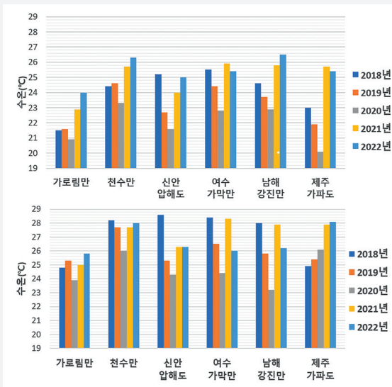
〈 주요 고수온 발생해역의 최근 5년간 월평균 표층수온 비교(7~8월) 〉
