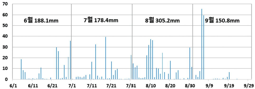
[그림 3-8-1] 월별 강수량 분포도
