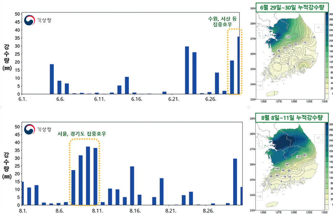
[그림 2-1-12] (위) 6월 강수량 일별 시계열과 6월 29일~30일 누적강수량(mm) 분포도
