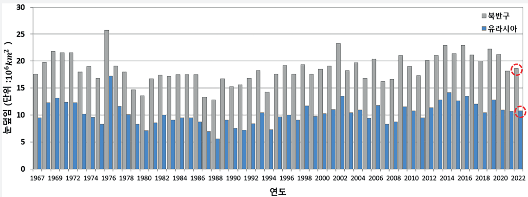
[그림 2-3-5] 1967~2022년 10월 북반구 및 유라시아 대륙 눈덮임 면적 시계열 ※ 출처: 럿거스 대학교(Rutgers University Snow lab), 빨간 원: 2022년 10월
