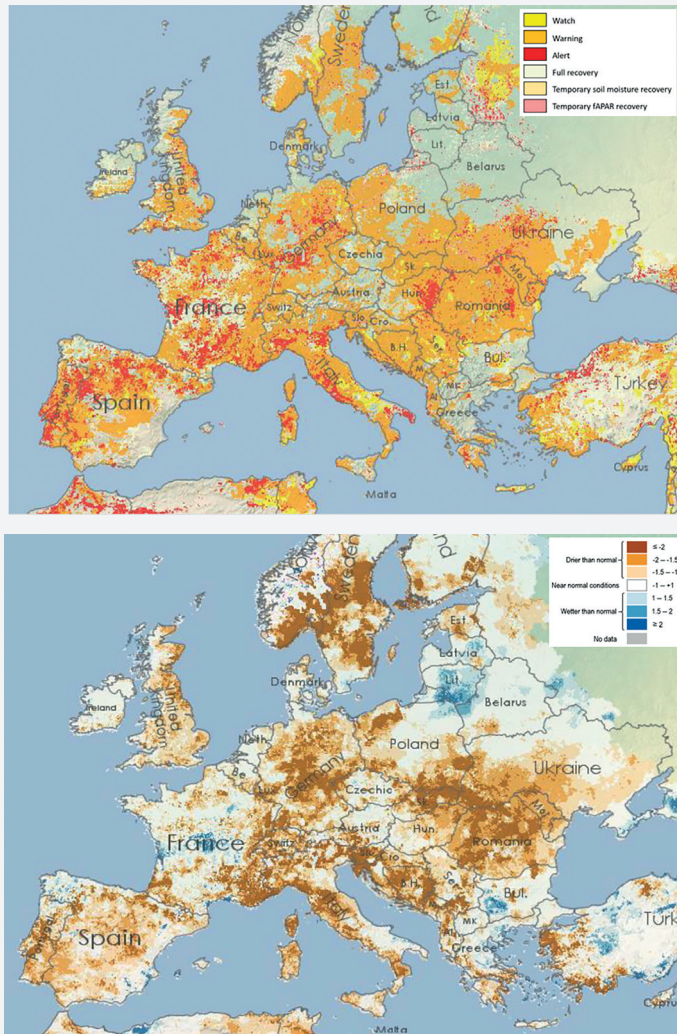
[그림 2-3-10] (상) 2022년 6월 복합가뭄지수(CDI: combined Drought Indicator), (하) 토양수분 편차 (출처:유럽연합 지구관측소)
