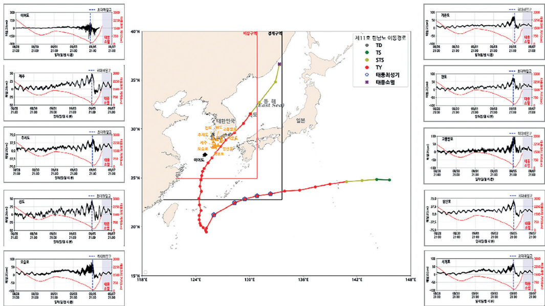
[그림 3-2-9] 제11호 태풍 ‘힌남노(HINNAMNOR)’ 통과시 주요 관측소에서의 해일고 시계열 (그림출처: 국립해양조사원 2022 Vol. 3 ‘태풍분석보고서’)
