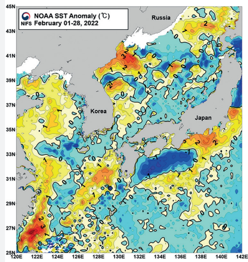
〈 '22년 2월 평균 평년대비 표면수온 편차 분포 〉
