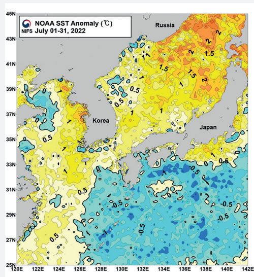
〈 '22년 7월 평균 평년대비 표면수온 편차 분포 〉
