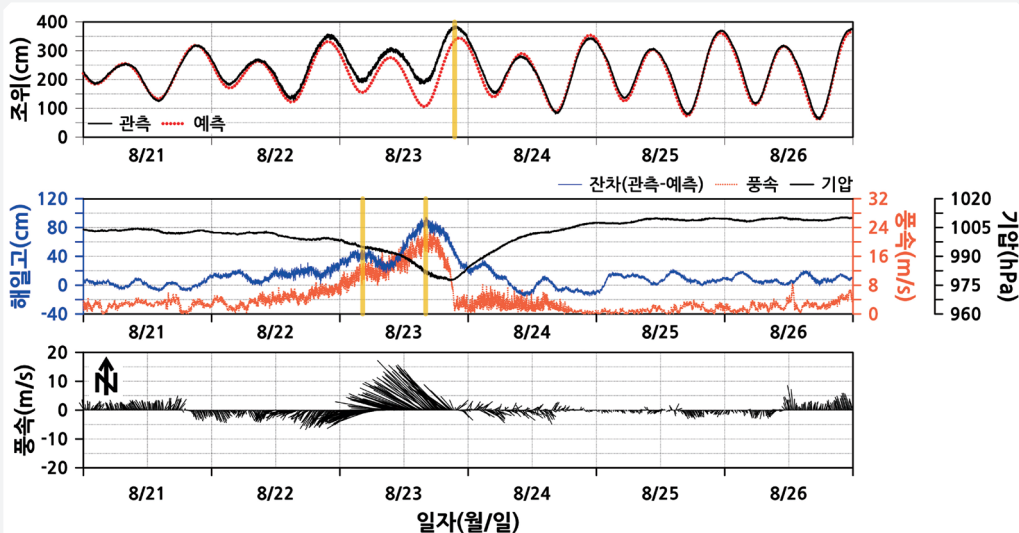
[그림 4-2-5] 제19호 태풍 ‘솔릭’ 통과시 진도 조위관측소에서의 해일고 및 기상자료 시계열 (그림출처 : 국립해양조사원 2018 Vol. 2 ‘태풍분석보고서’)
