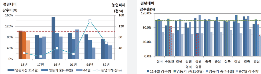
[그림 4-8-4] (왼쪽) 가뭄 발생년도와 평년대비 강수, (오른쪽) '18년 지역별 평년대비 강수량비교
