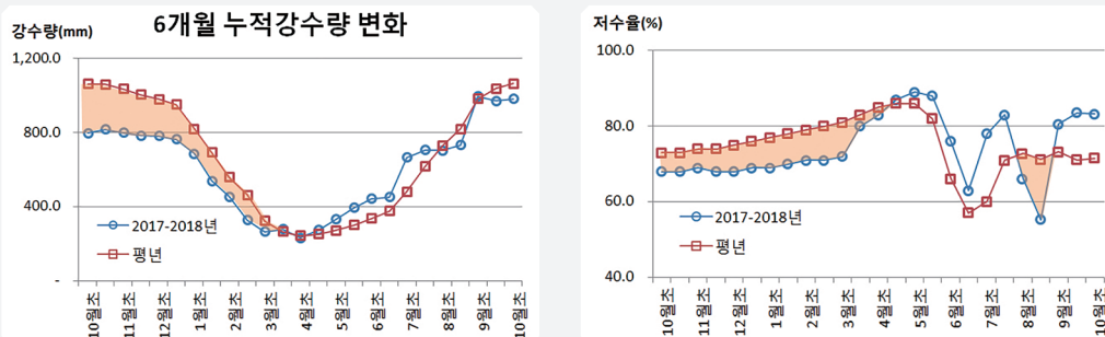
[그림 4-8-5] (왼쪽) 6개월 누적 강수량 변화, (오른쪽) 농업 저수지 저수율 변화
