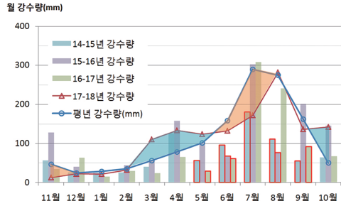
[그림 4-8-3] (왼쪽) '17~'18년 전국 연 평균 강수량 비, (오른쪽) '18년 전국 평균 강수량 비교
