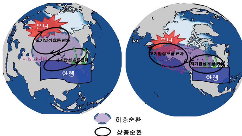
[그림 3-2-5] (왼쪽)바렌츠-카라 해 및 (오른쪽)척치 해의 북극해빙면적이 적은 경우, 동아시아 지역과 북미 지역의 한파 발생에 미치는 영향에 대한 모식도 (그림출처 : 포항공대 기후시스템연구실)
