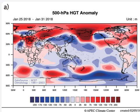
[그림 3-2-23] 2018년 1월25일부터 31까지 평균된 a) 500mb 지위고도 와 b) 바람장 평년 편차도 (그림출처 : www.apcc21.org)
