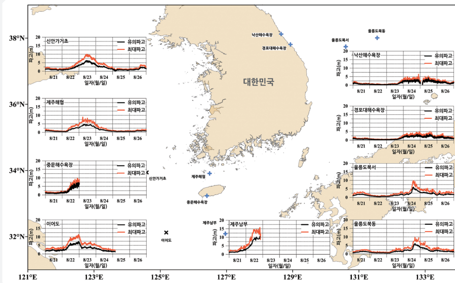
[그림 4-2-8] 제19호 태풍 ‘솔릭’ 통과시 해양과학기지 및 해양관측부이에서의 최대파고 및 유의파고 (그림출처 : 국립해양조사원 2018 Vol. 2 ‘태풍분석보고서’)
