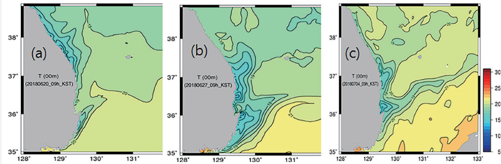
[그림 4-2-19] 국립수산물학원 동해 냉수대 예측정보시스템을 통한 2018년 (a) 6월 20, (b) 6월 27일, (c) 7월 4일 냉수대 예측 결과 (그림출처 : 국립수산물학원)
