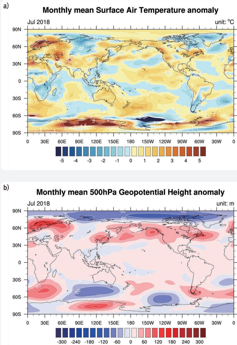
[그림 3-2-11] 2018년 7월 동안 a) 지표온도와 b) 500hPa 지위고도의 평년 편차도 (그림출처 : http://www.apcc21.org )
