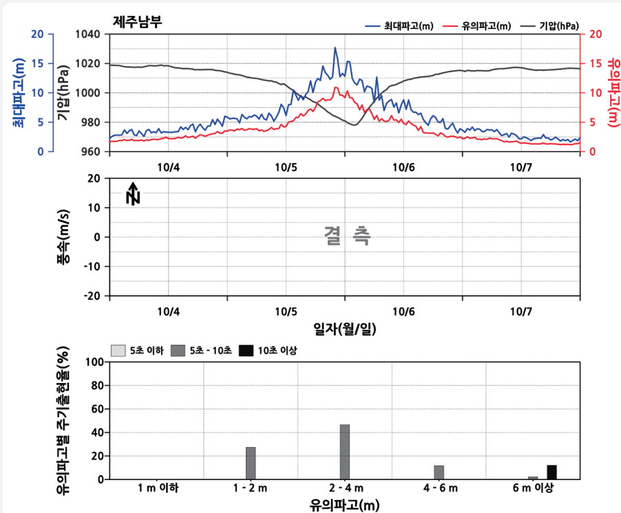
[그림 4-2-11] 제25호 태풍 ‘콩레이’ 통과시 제주남부 해양관측부이의 기상자료 시계열과 파고 분석 결과 (그림출처 : 국립해양조사원 2018 Vol. 3 ‘태풍분석보고서’)
