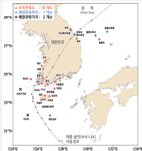
[그림 4-2-1] 2018년 제19호 태풍 ‘솔릭(SOULIK)’의 이동 경로(그림출처 : 기상청) 및 영향권에 속한 주요 관측소 위치도(그림출처 : 국립해양조사원 2018 Vol. 2 ‘태풍분석보고서’)
