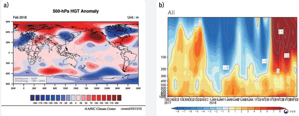
[그림 3-2-19] a) 2018년 2월 500 hPa 지위고도 평년 편차도(그림출처 : http://www.apcc21.org )와 b) 2017년 12월부터 2018년 2월까지 북극 지역에서 평균된 연직 기온 평년 편차도 (그림출처 : http://co-anal.kma.go.kr )
