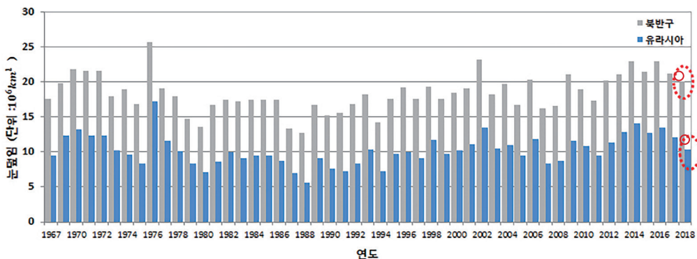
[그림 3-2-8] 10월 북반구 및 유라시아 대륙 눈덮임 면적 시계열 (빨간 원 : 2018년 10월)
