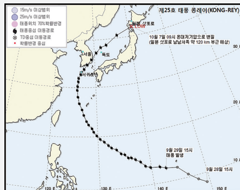
[그림 3-1-19] 2018년 우리나라에 상륙한 태풍 진로도
