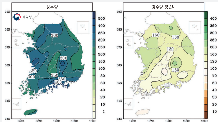
[그림 3-1-7] 장마 기간(6.19.~7.11.) 강수량(mm) 및 강수량 평년비(%) 분포도
