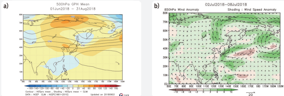
[그림 3-2-15] a) 2018년 여름철(6월-8월) 평균 500 hPa 지위고도 평년 편차도, b) 2018년 7월 2일부터 8일까지 평균된 850 hPa 바람장(벡터)과 속력(색갈) 평년 편차도 (그림출처 : http://co-anal.kma.go.kr )
