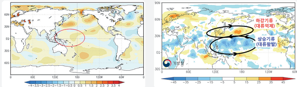
[그림 3-1-15] 7월 (왼쪽)해수면온도편차(빨강/파랑 채색: 평년보다 높/낮은 해수면온도)와 (오른쪽)상향장파복사 3) 편차(빨강/파랑 채색: 평년보다 대류(상승기류) 억제/활발
