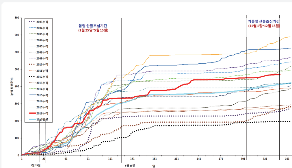
[그림 4-3-2] 2018년 일자별 누적 산불 건수 변화
