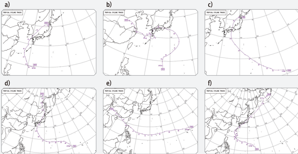
[그림 3-2-14] 2018년 7월에서 8월에 일본, 필리핀, 중국에 피해를 입힌 태풍의 이동 경로 모식도. a) 제7호 태풍 ‘쁘라빠룬’, b) 제12호 태풍 ‘종다리’, c) 제20호 태풍 ‘시마론’, d) 제21호 태풍 ‘제비’, e) 제22호 태풍 ‘망쿳’, f) 제24호 태풍 ‘자미’ (그림출처 : https://www.jma.go.jp )
