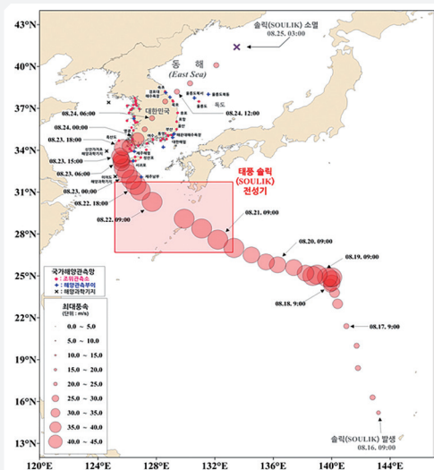
[그림 4-2-1] 2018년 제19호 태풍 ‘솔릭(SOULIK)’의 이동 경로(그림출처 : 기상청) 및 영향권에 속한 주요 관측소 위치도(그림출처 : 국립해양조사원 2018 Vol. 2 ‘태풍분석보고서’)
