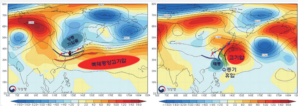
[그림 3-1-11] 500hPa 지위고도 편차 분포도 (왼쪽)상층 기압골의 영향기간(2018년 6월 26일~28일), (오른쪽)태풍 ‘쁘라삐룬’의 영향기간(2018년 7월 1일~2일)
