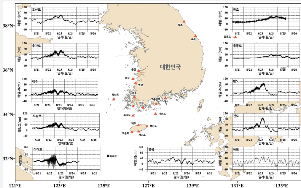
[그림 4-2-4] 제19호 태풍 ‘솔릭’ 통과시 주요 관측소에서의 해일고 시계열 (그림출처 : 국립해양조사원 2018 Vol. 2 ‘태풍분석보고서’)
