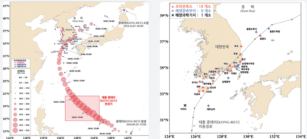
[그림 4-2-2] 2018년 제25호 태풍 '콩레이(KONG-REY)'의 이동 경로(그림출처: 기상청) 및 영향권에 속한 주요 관측소 위치도(그림출처: 국립해양조사원 2018 Vol. 3 '태풍분석보고서')
